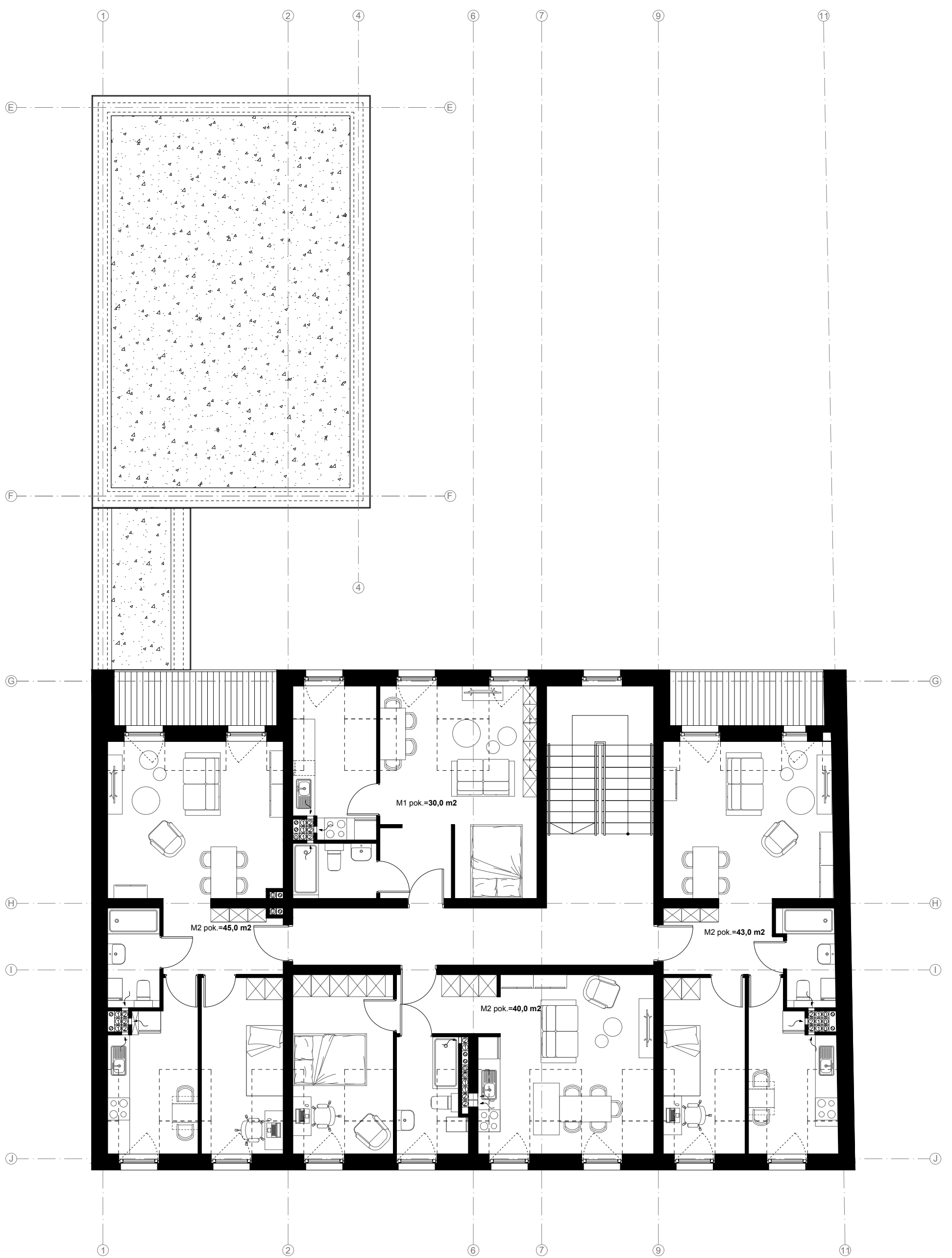
BUDYNEK A i B - RZUT PODDASZA 1:100
