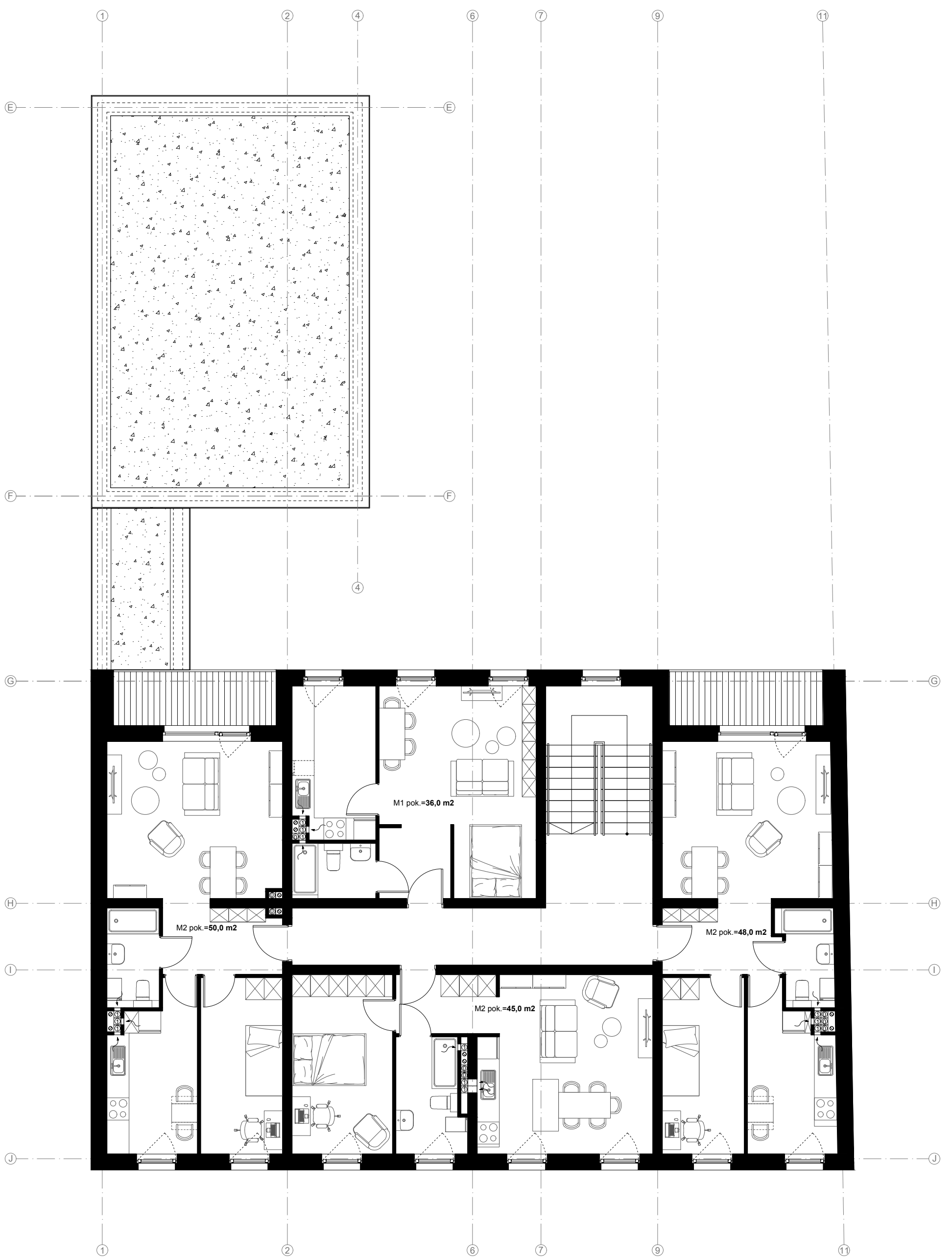
BUDYNEK A I B - RZUT I PIĘTRA 1:100
