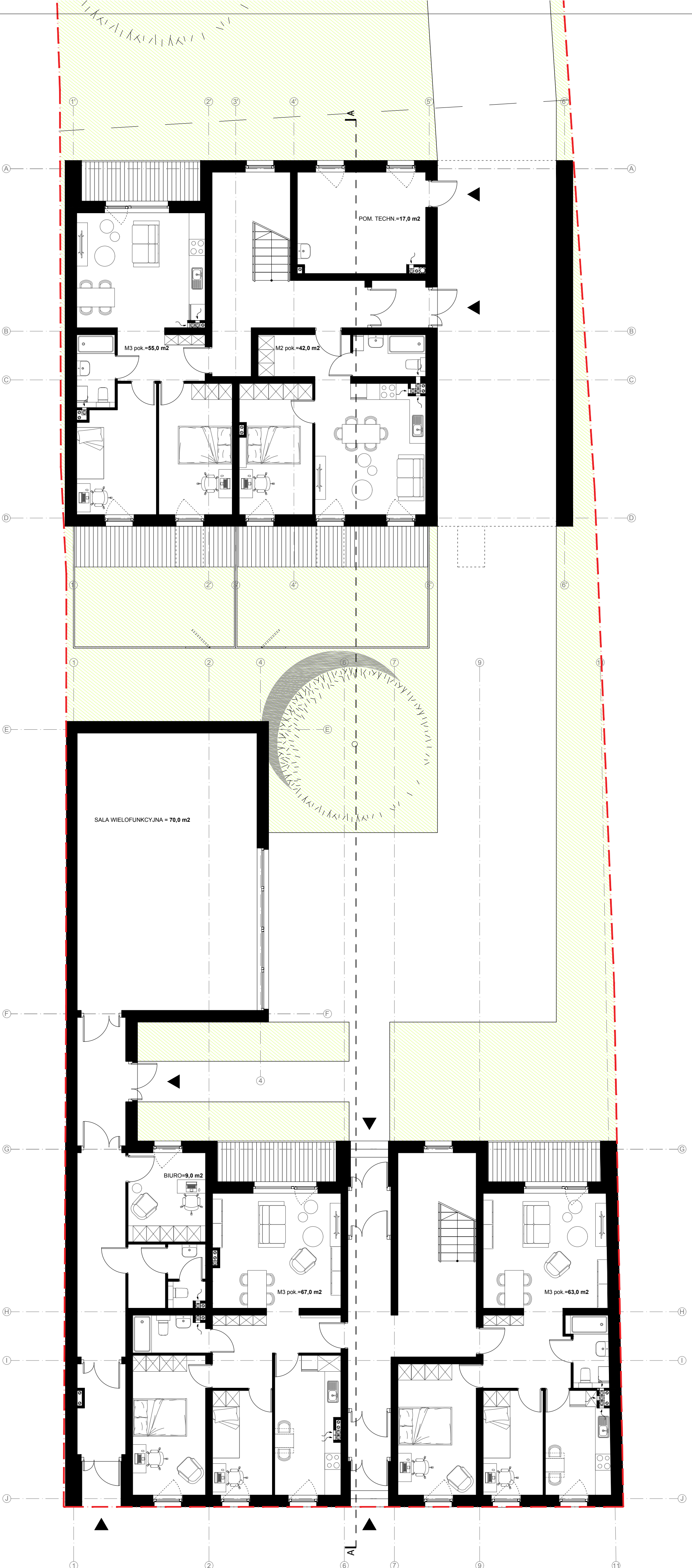
BUDYNEK A i B - RZUT PARTERU 1:100
